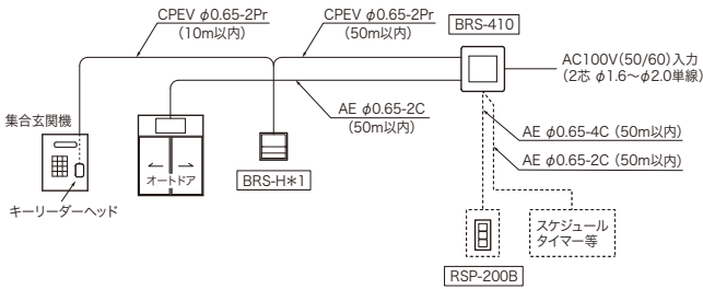
オートドアの場合
