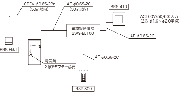
電気錠の場合
